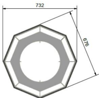
9004 Ø700 H400 or H600
